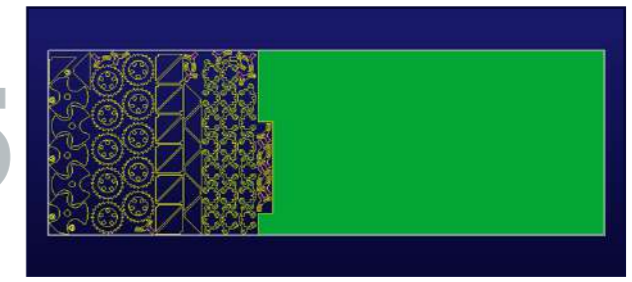
A sinistra tutti i pezzi sono stati nestizzati, a destra la porzione di lamiera raffigurata in verde è la rimanenza che ritornerà in magazzino per i lavori successivi.
